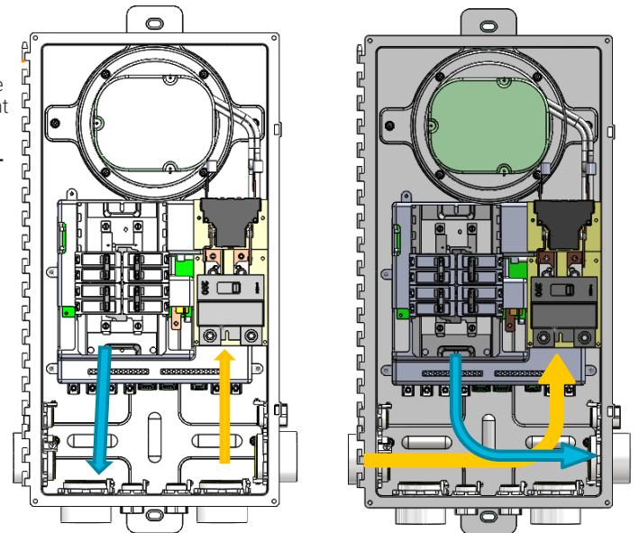
Conduit guidance - bottom entry
